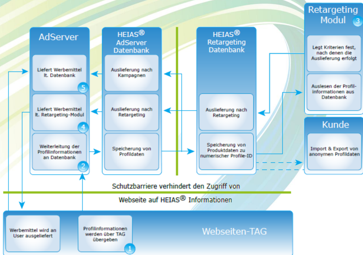
Abbildung 1: Prozessdarstellung Werbemittelauslieferung mit HEIAS®
